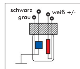
4 Kabel
