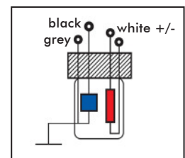
4 cables
