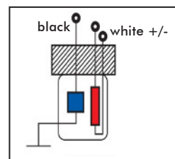
3 cables
